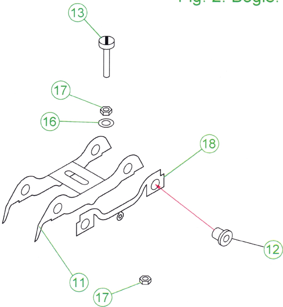
Fig. 2. Bogie.
